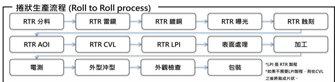
圖 2 軟板基礎製造流程
