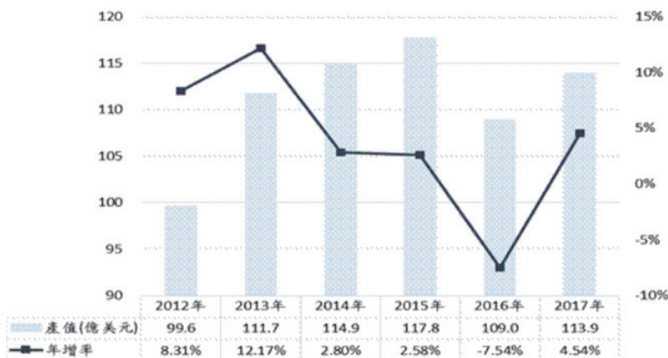
圖二 全球軟性印刷電路板業產值及年增率走勢
