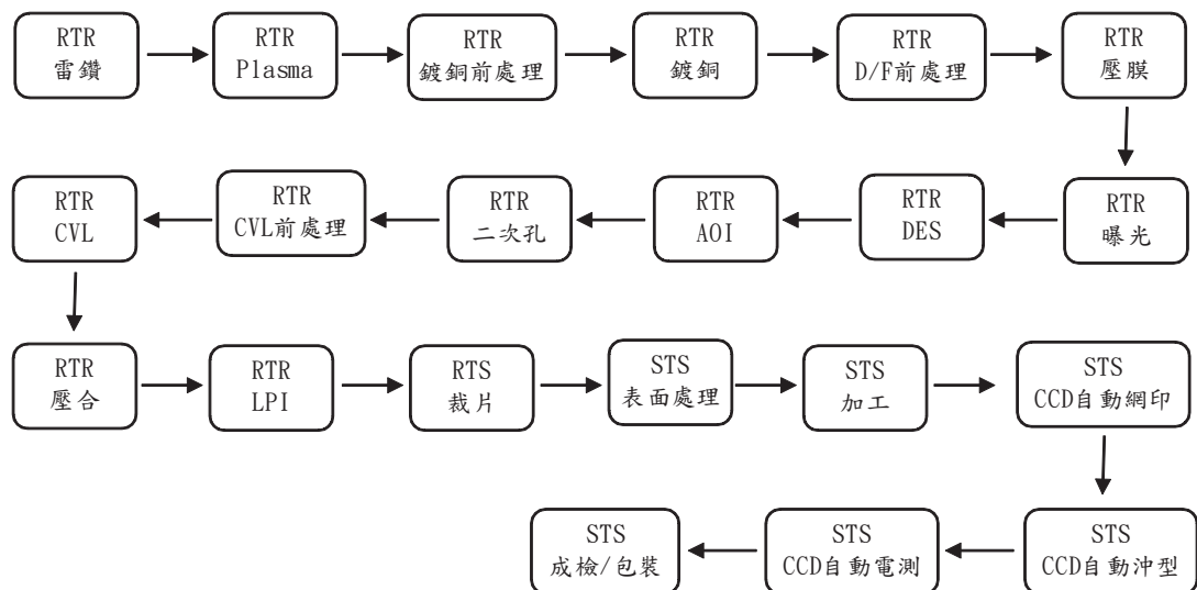
圖 2 軟板基礎製造流程
